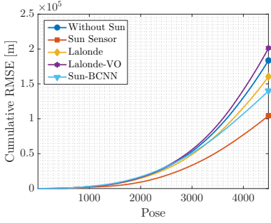
(d) 00: Translational CRMSE
