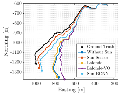
(b) 01: VO trajectories (EN-plane)
