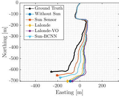
(a) 00: VO trajectories (EN-plane)
