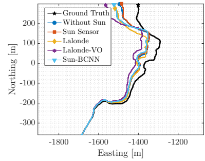
(c) 05: VO trajectories (EN-plane)
