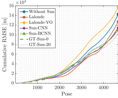
(d) 02: Translational CRMSE (EN-plane)
